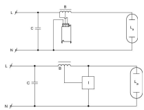
Technische Daten Philips HID-Hochspannung BSN 1000 L78 230/240V 50Hz HP-257
